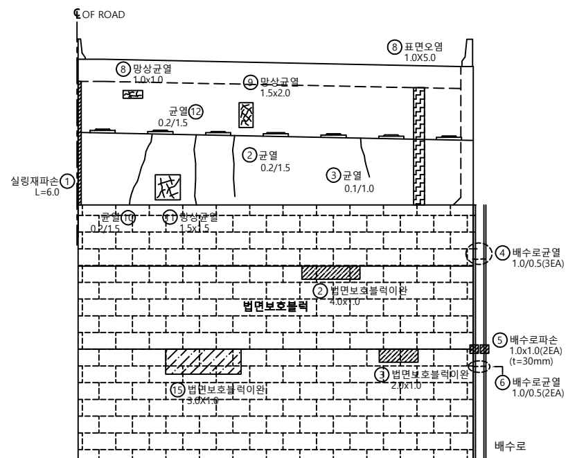
정 면 도
